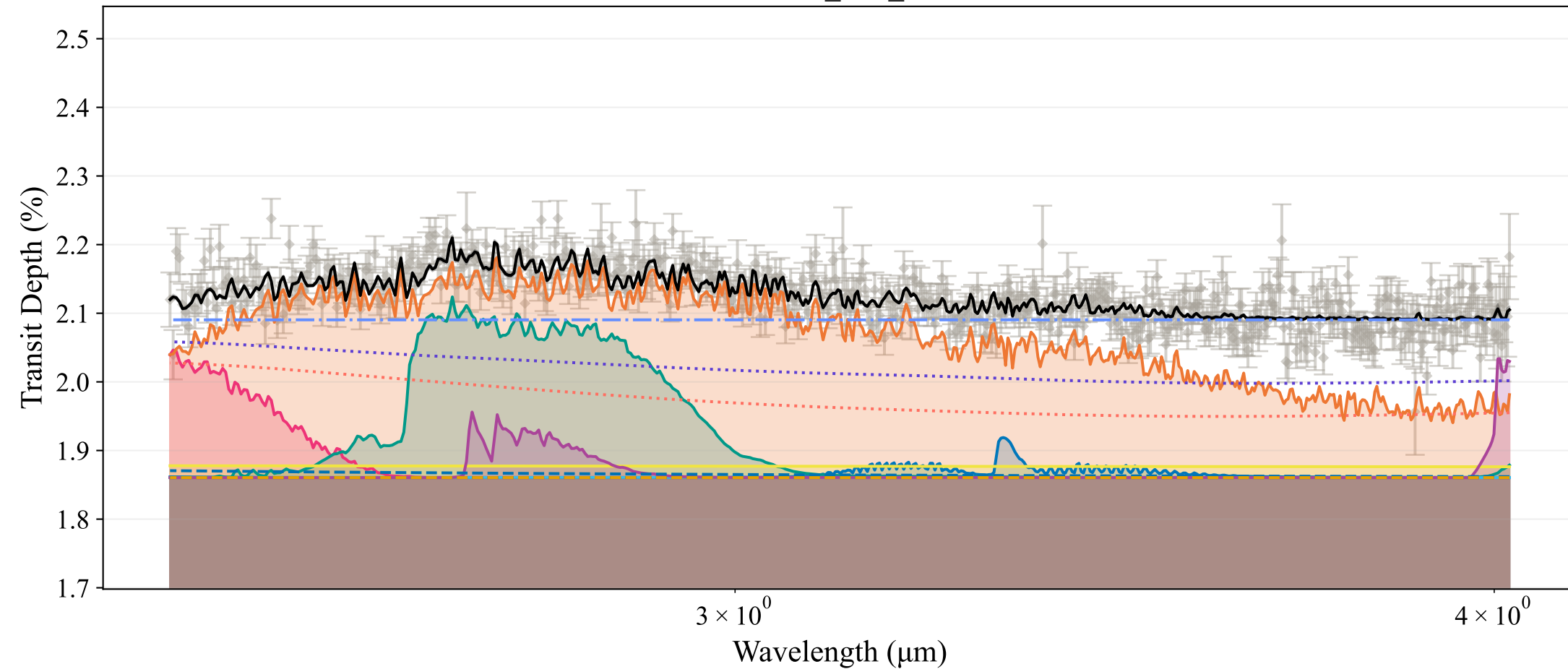
nircam_SiO_iso
